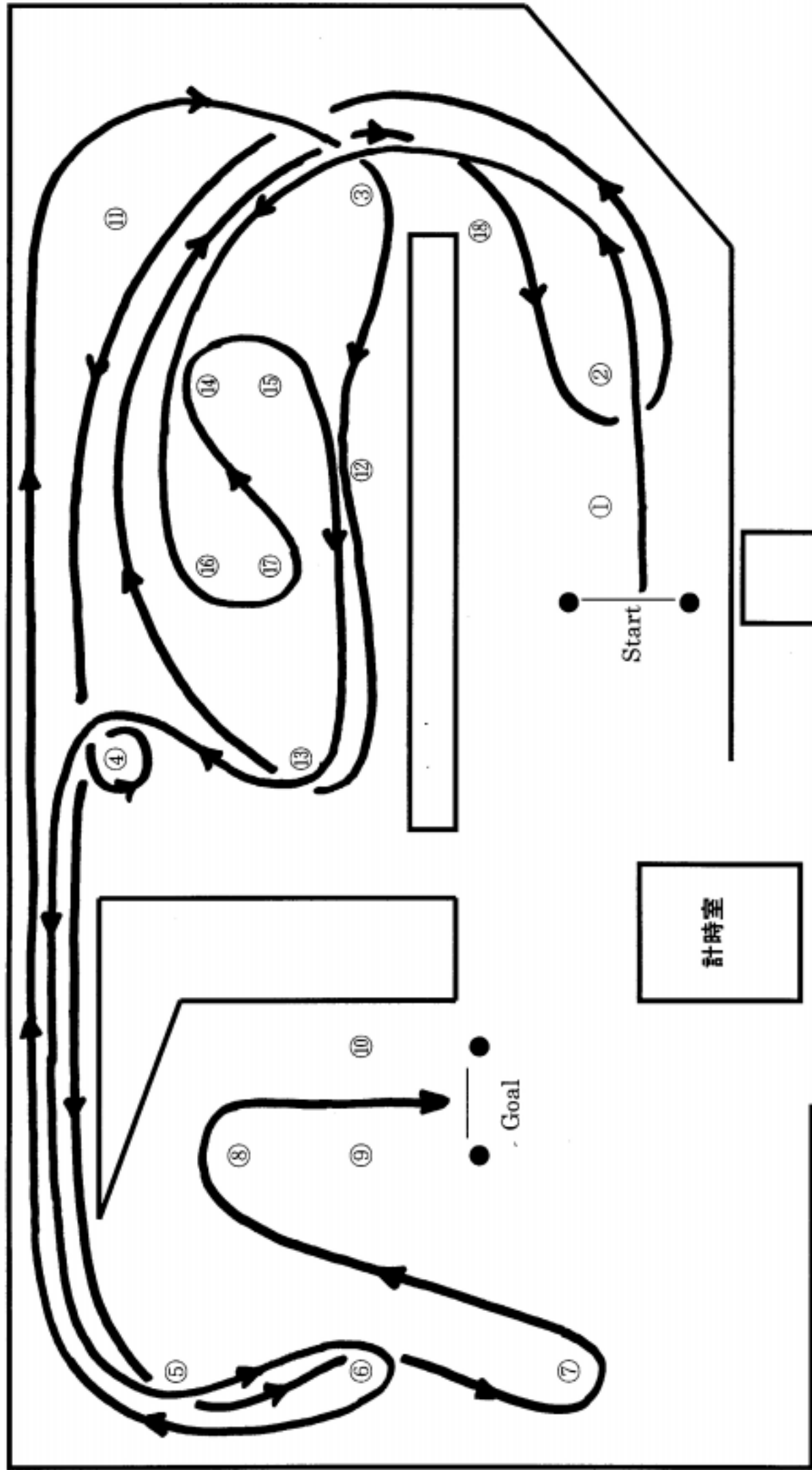
99JMRC 茨城ジムカーナシリーズ第2戦 ICC.S コース図 (Designed by BaneG)
